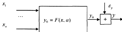
Рис. 1.1. Модель процесса в виде «черного ящика». Обозначения: x_1, \dots, x_n – истинные значения вектора входных переменных; y_0 , y – значения детерминированной и случайной составляющих выходной переменной моделируемого процесса; \varepsilon_y – ненаблюдаемые внутренние аддитивные «шумы»; a – вектор параметров.
