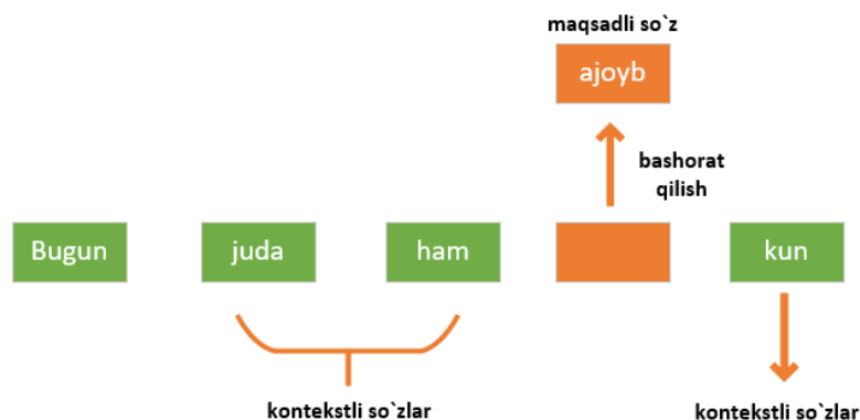
1-rasm. CBOW metodi sxemasi
